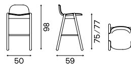
Stool
